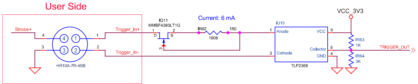
그림 7-4 Input Schematic
