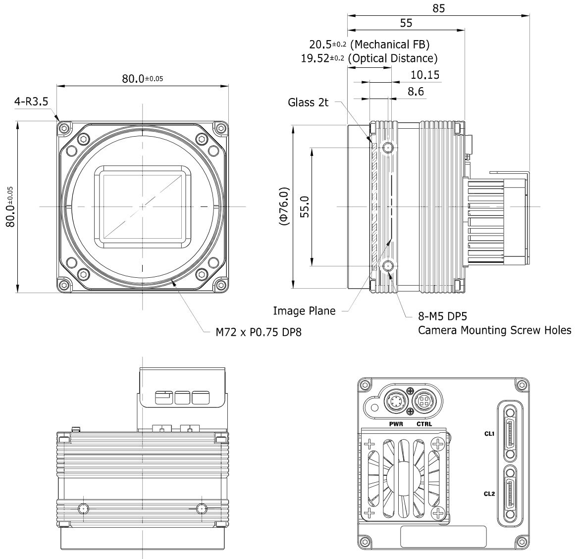
그림 5-3 VC-103MC-M/C7I Mechanical Dimension
