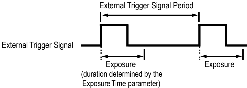
그림 8-4 Timed Exposure Mode
