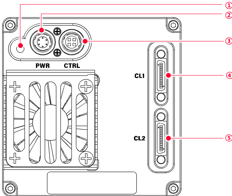
그림 7-1 VC-103MC-M/C7I Back Panel
