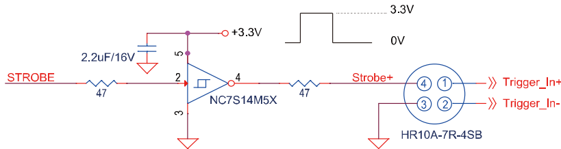
그림 7-5 Output Schematic
