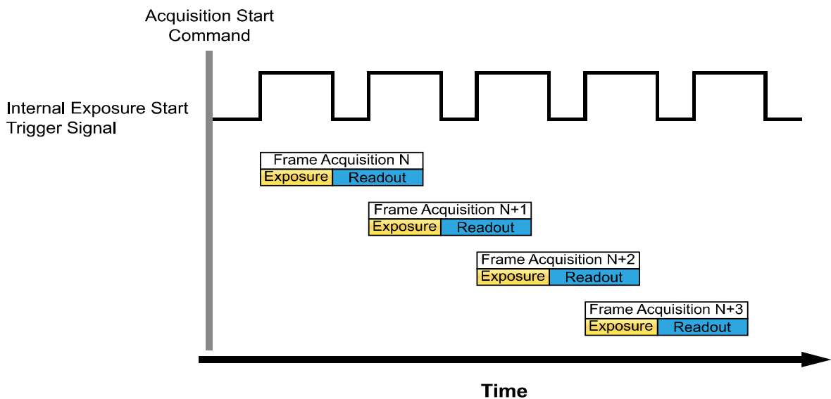
그림 8-7 Overlapped Exposure and Readout
