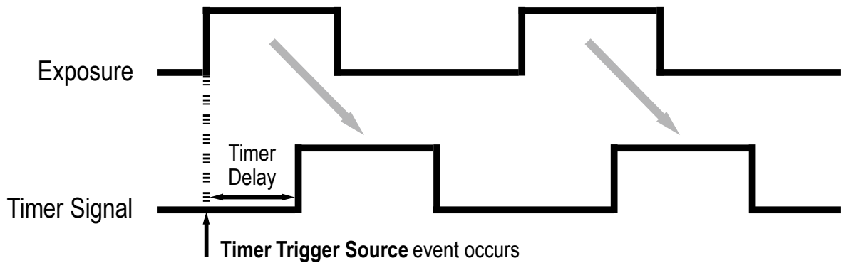
그림 9-16 Timer Signal
