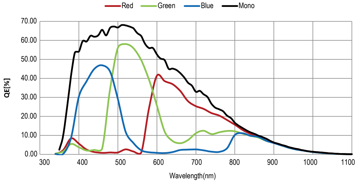
그림 5-2 VC-103MC-M/C7I Spectral Response
