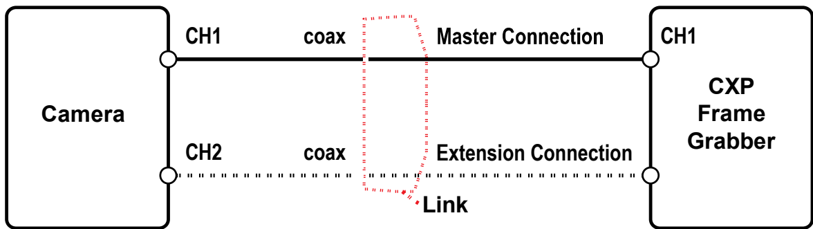
그림 9-4 CXP Link Configuration
