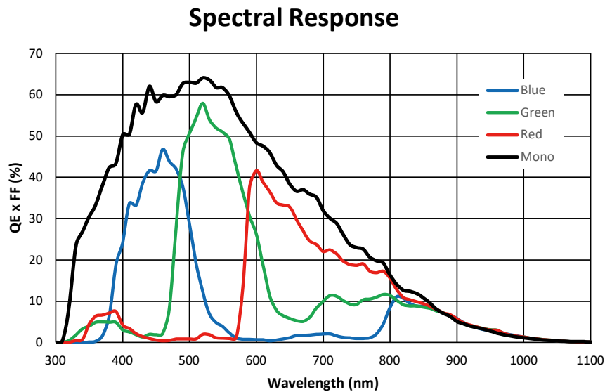
그림 5-3 VC-18MX2 시리즈의 Spectral Response
