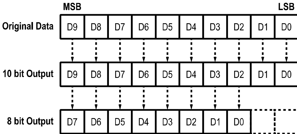
그림 9-5 VC-5/9/18MX2 시리즈 Pixel Format
