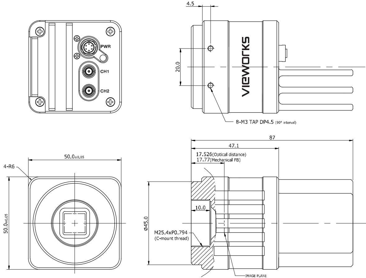
그림 5-4 VC-5/9/18MX2 시리즈 Mechanical Dimension
