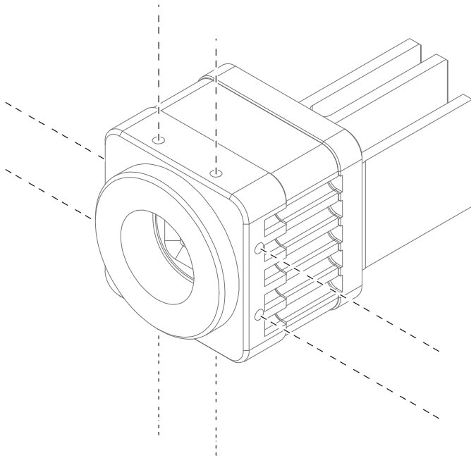
그림 5-6 VC-5/9/18MX2 시리즈 제품을 거치할 때 고정나사 위치
