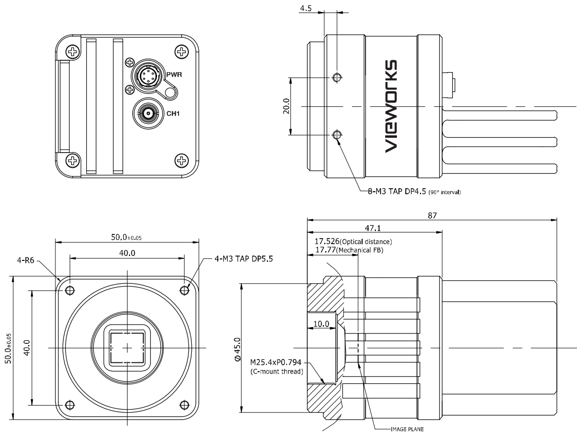
그림 5-5 VC-9MX2-M120I00의 Mechanical Dimension
