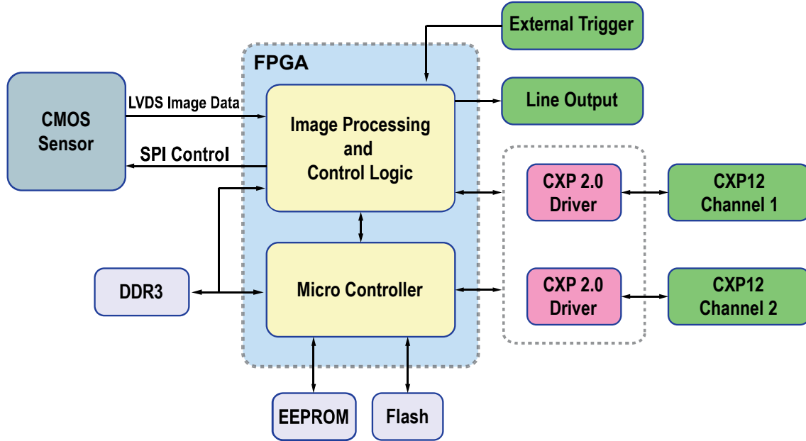
그림 5-1 Camera Block Diagram
