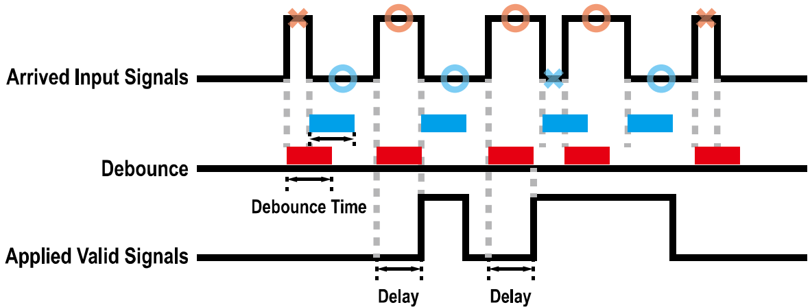
그림 9-13 Debounce
