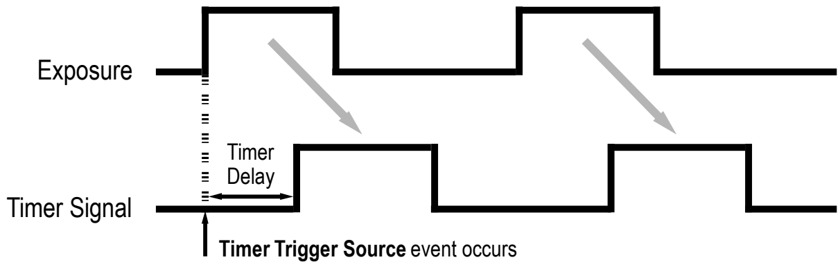
그림 9-14 Timer Signal
