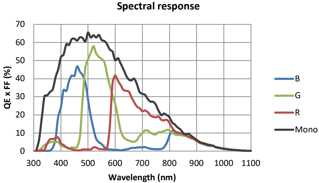
그림 5-2 VC-5/9MX2 시리즈의 Spectral Response
