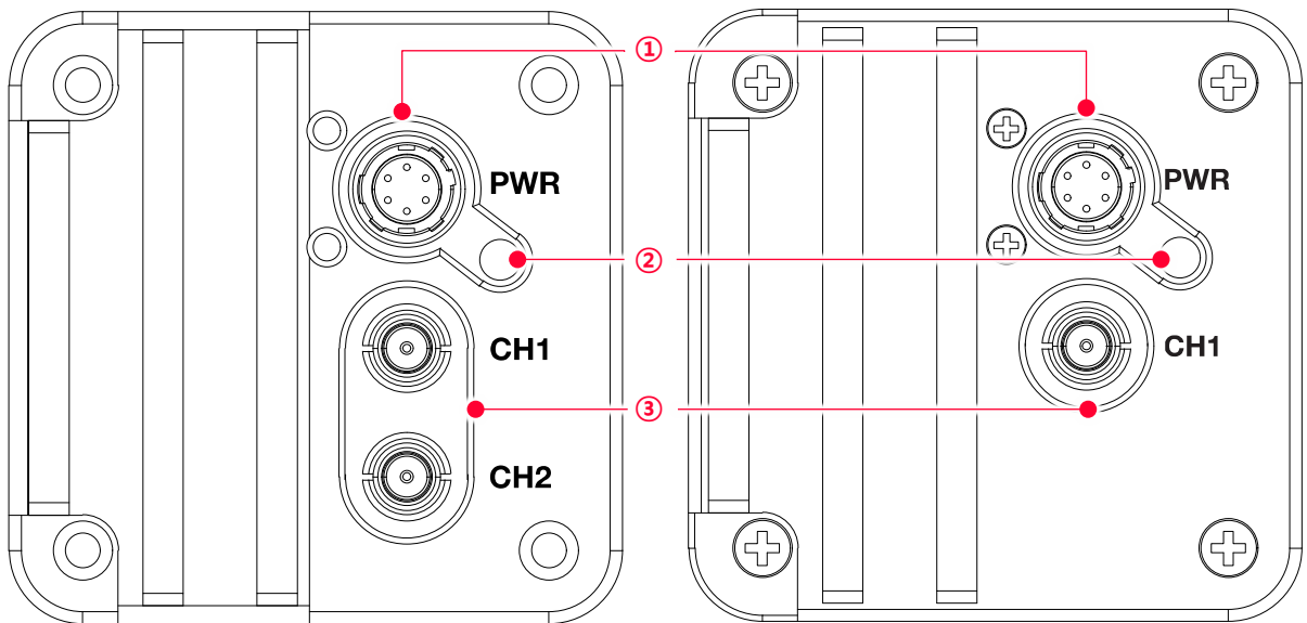
그림 7-1 VC-5/9/18MX2 시리즈 Back Panel
