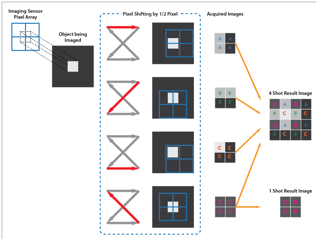
Figure 9.10 Pixel Shifting 출력 영상과 기본 영상과의 비교
