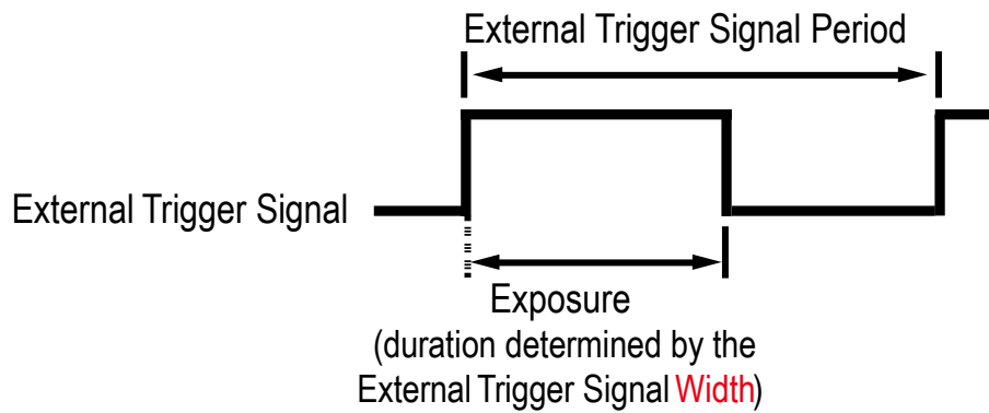
그림 8-5 Trigger Width Exposure Mode
