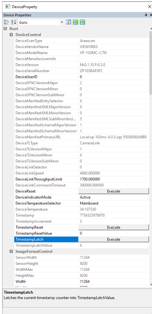
그림 10-3 Device Property
