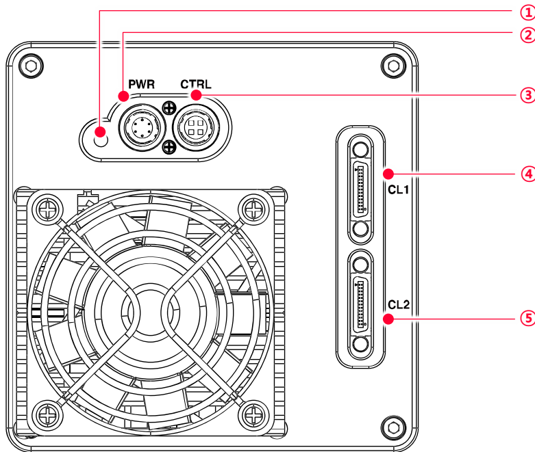
그림 7-1 VP-103MC-M/C7I Back Panel
