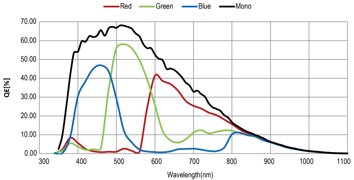
그림 5-2 VP-103MC-M/C7I Spectral Response
