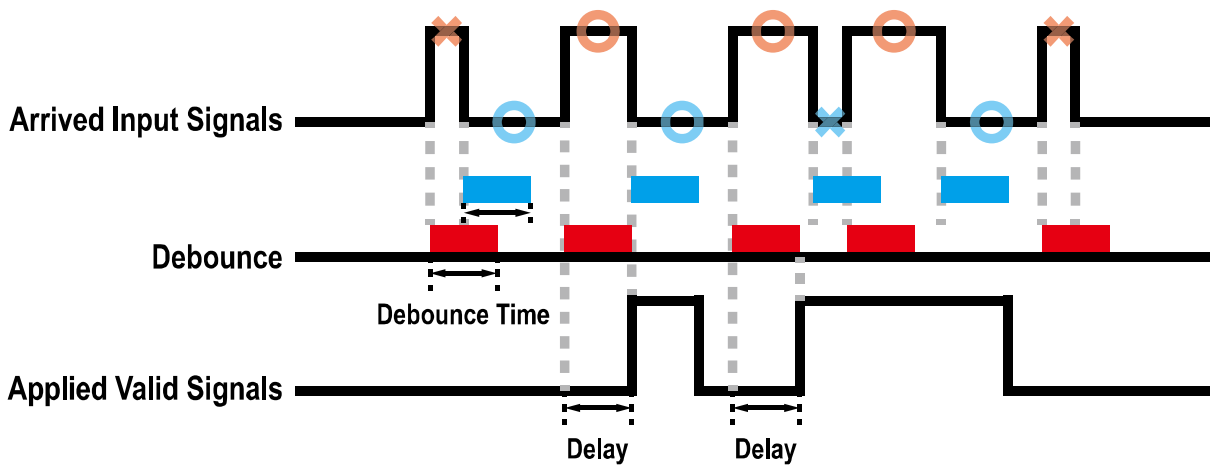
그림 9-15 Debounce
