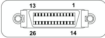
그림 5-1 Camera Block Diagram Camera Link 커넥터
