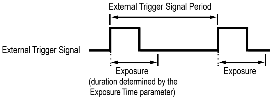
그림 8-3 Timed Exposure Mode
