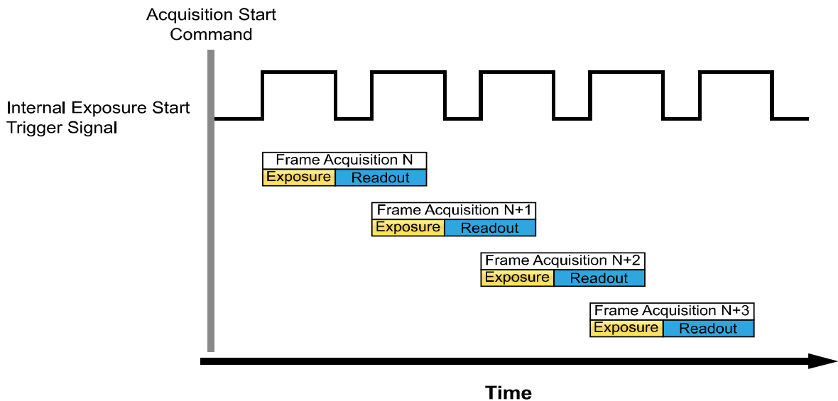
그림 8-6 Overlapped Exposure and Readout
