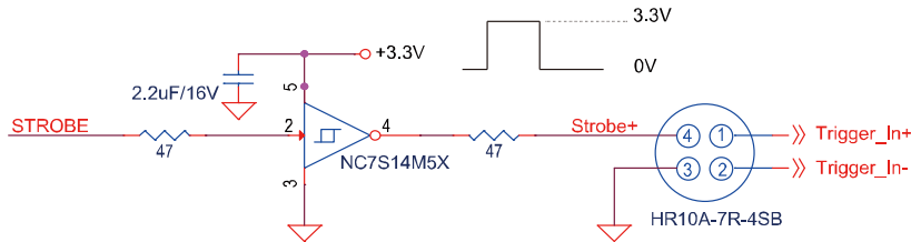
그림 7-4 Output Schematic
