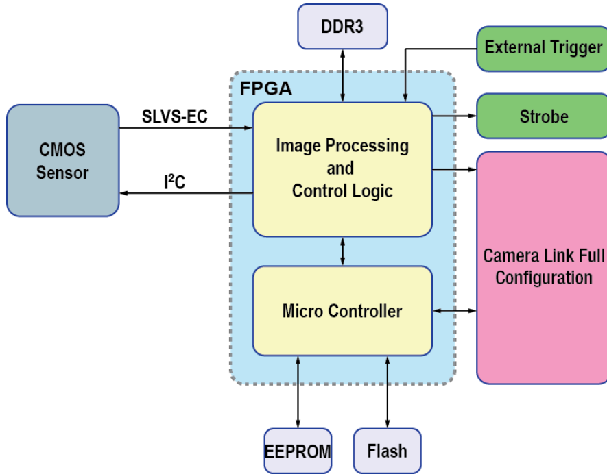
그림 5-1 Camera Block Diagram
