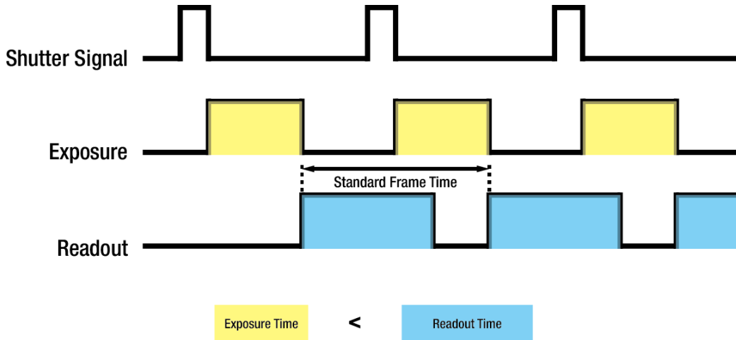
Figure 8.6 Exposure Time이 Readout Time보다 짧을 때
