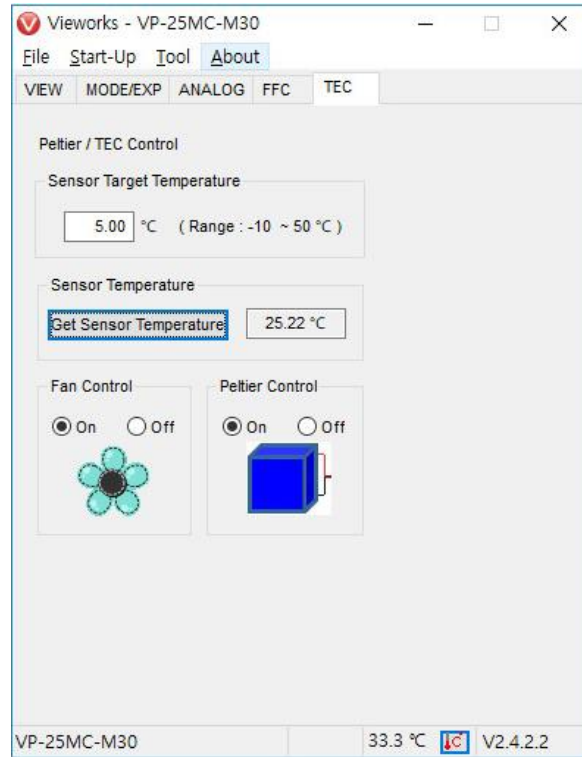
Figure 10.11 TEC Tab
